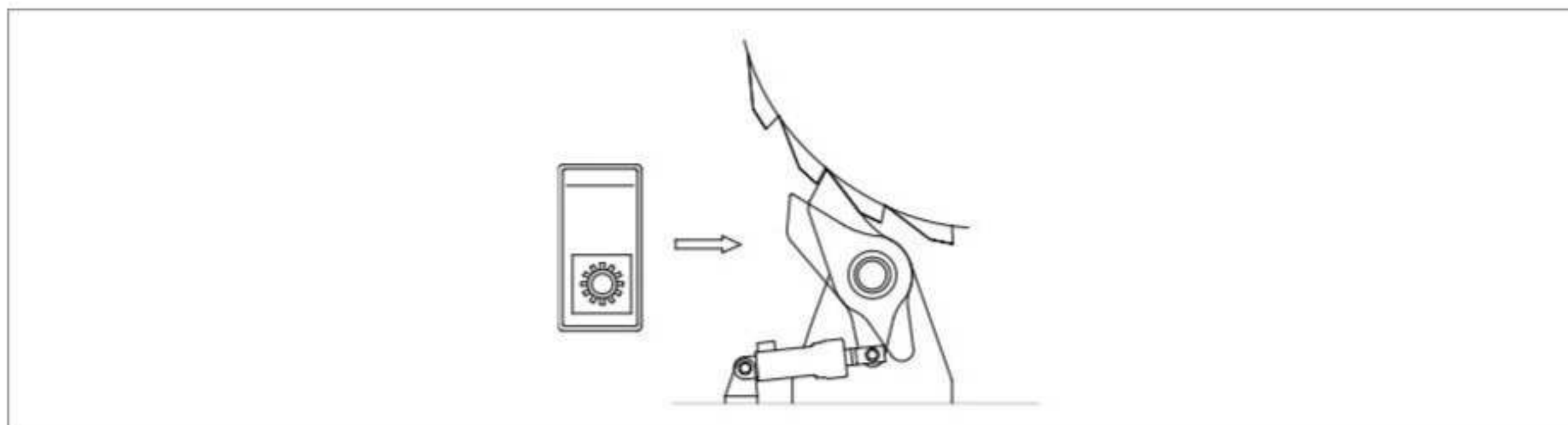
Рисунок 4-32 Храповой механизм стреловой лебедки
