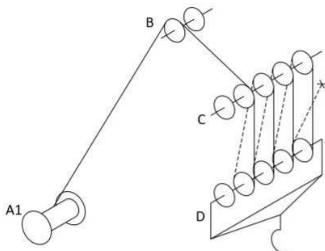
Рисунок 4-37 Схема запасовки каната (крюковая подвеска 100 т, кратность запасовки 8)
