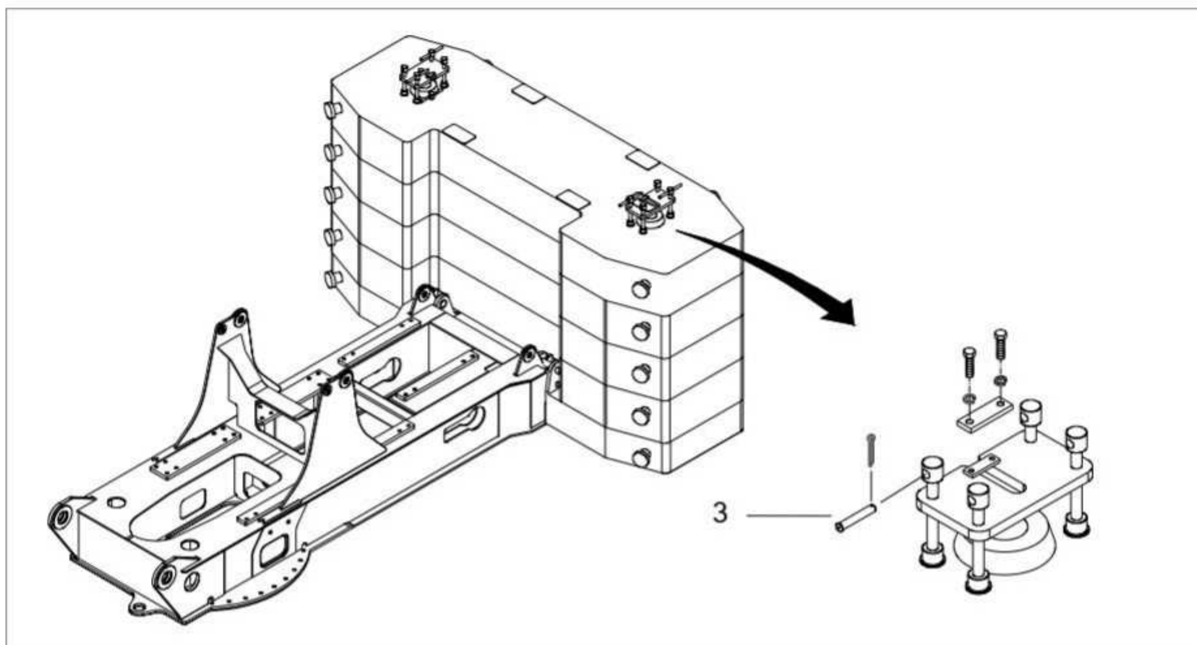
Рисунок 5-8 Закрепление плит противовеса цепью
