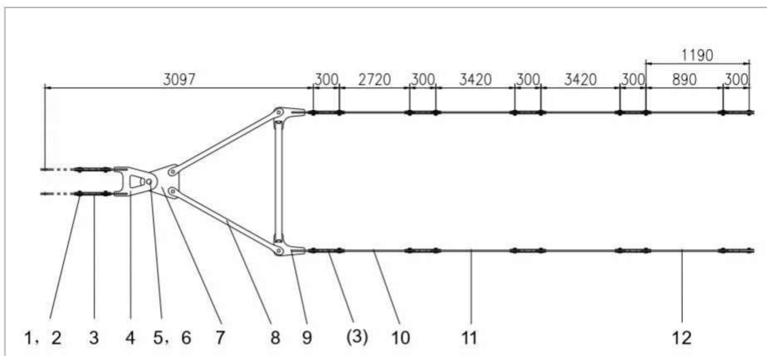
Рисунок 5-11 Соединение тяговых пластин задней растяжки жесткого гуська
