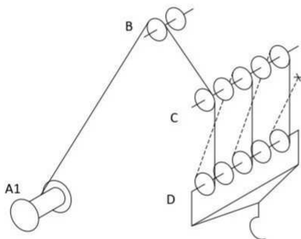
Рисунок 4-38 Схема запасовки каната (крюковая подвеска 100 т, кратность запасовки 6)
