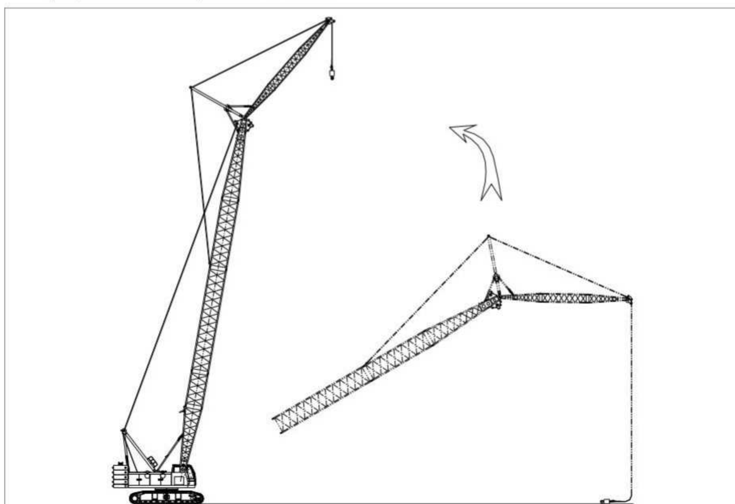
Рисунок 5-25 Подъем стрелы с жестким гуськом
