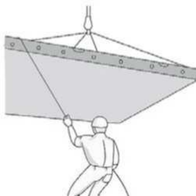
Рисунок 3-4 Действие оттяжки
