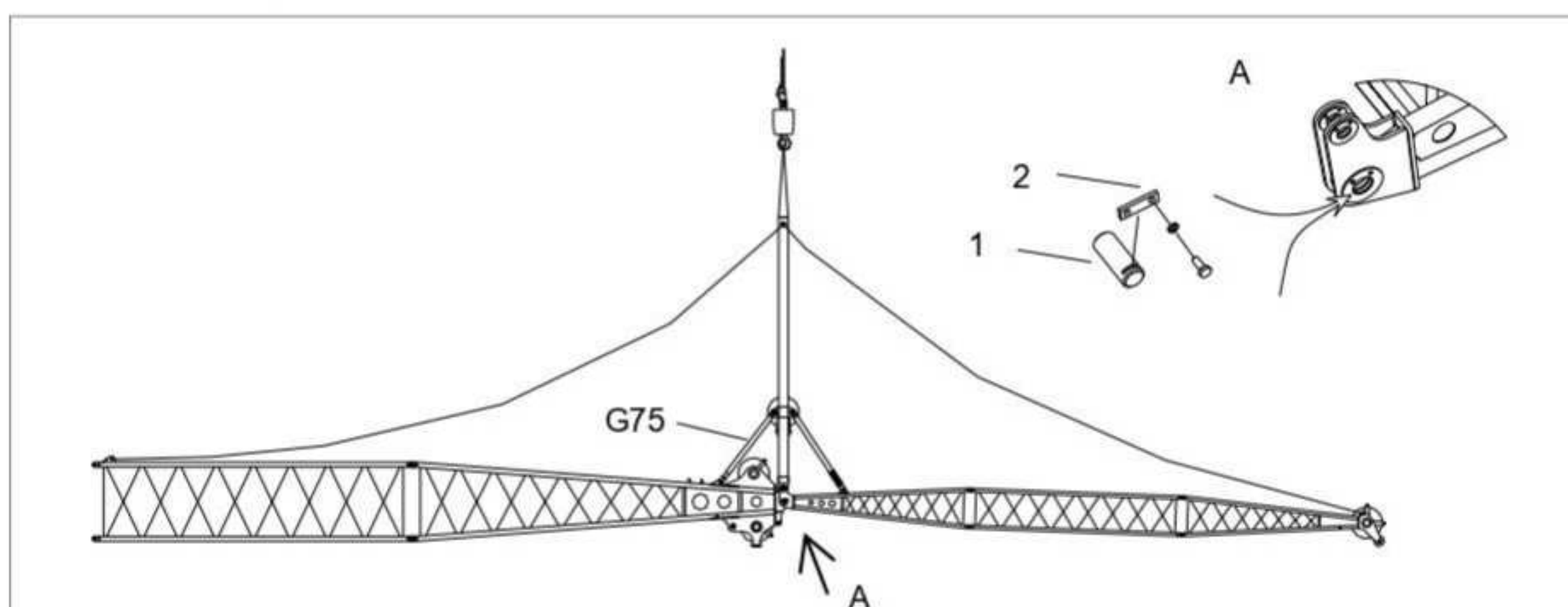
Рисунок 5-22 Монтаж стойки и передней растяжки жесткого гуська
