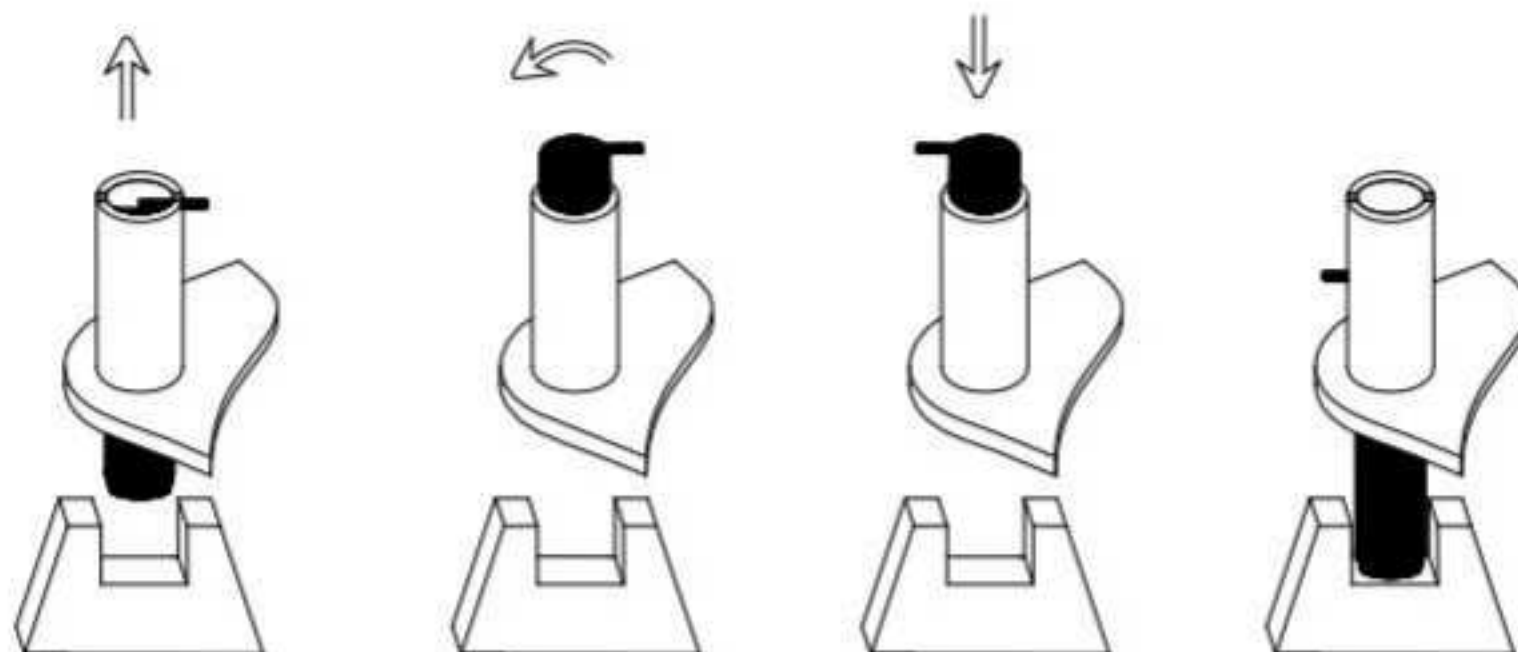
Рисунок 4-34 Фиксация поворотной платформы
