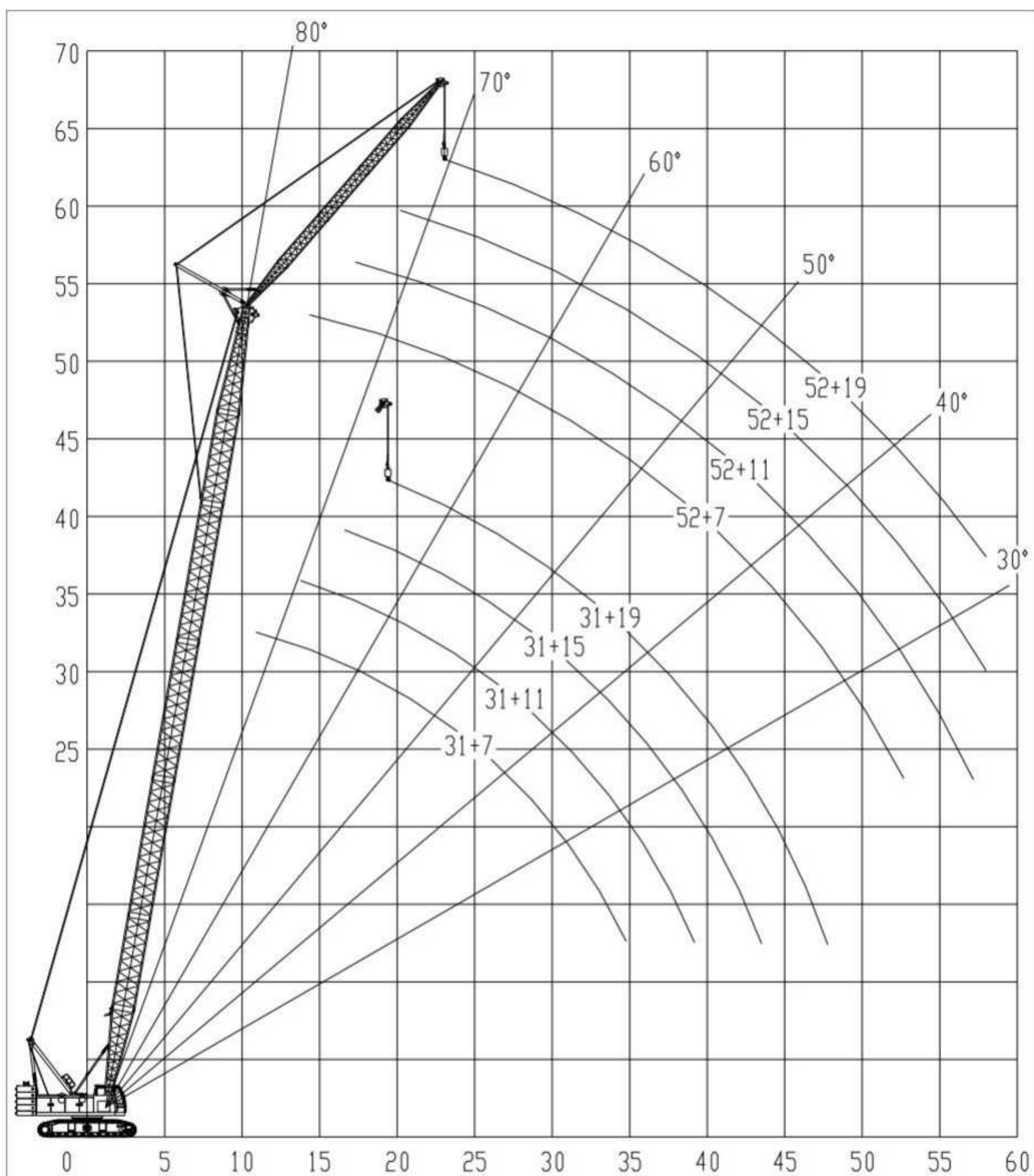
Рисунок 2-8 Диаграмма грузовысотных характеристик (SF-1, SF-2, 30°)
