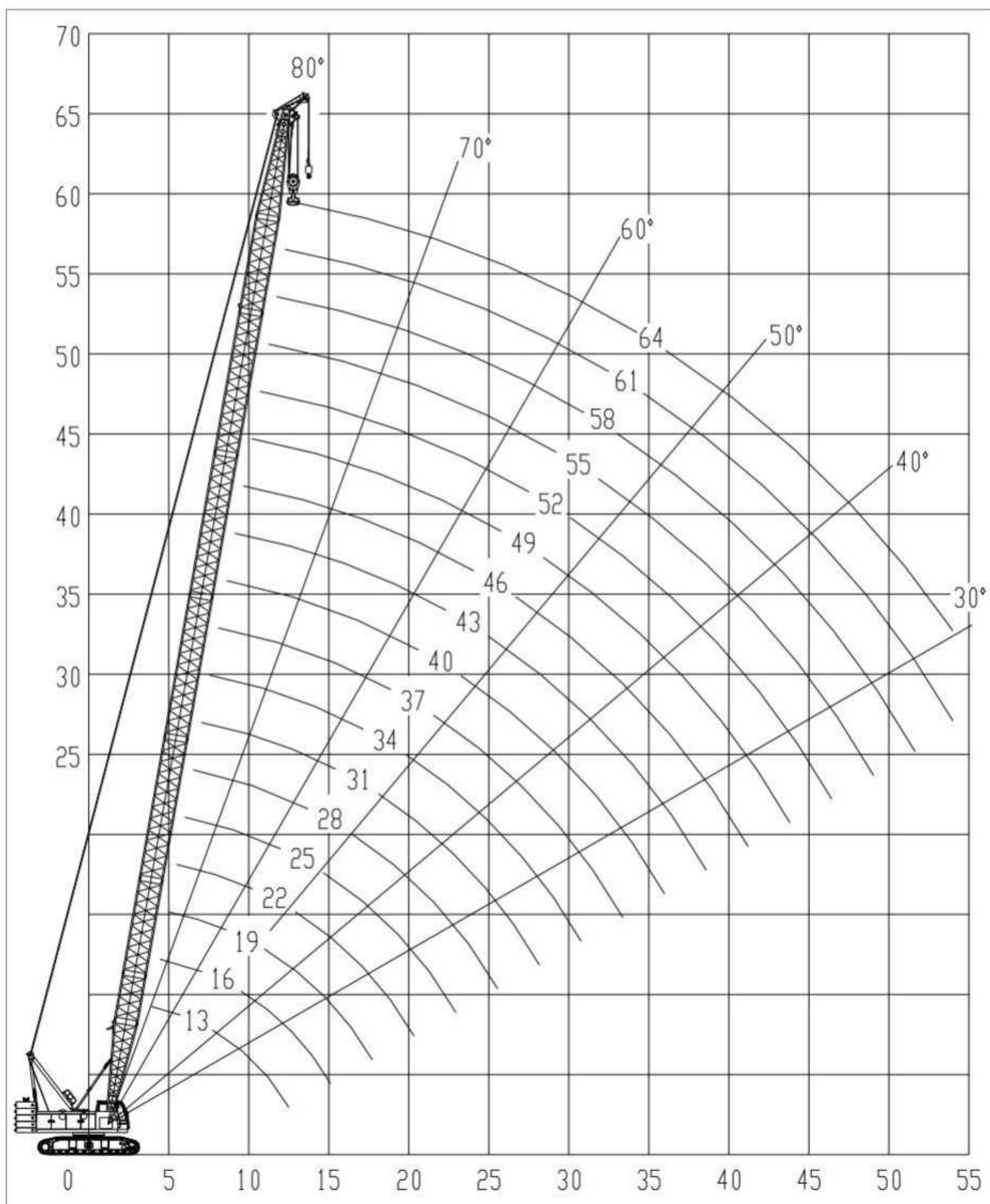
Рисунок 2-6 Диаграмма грузовысотных характеристик (S-1, S-2)
