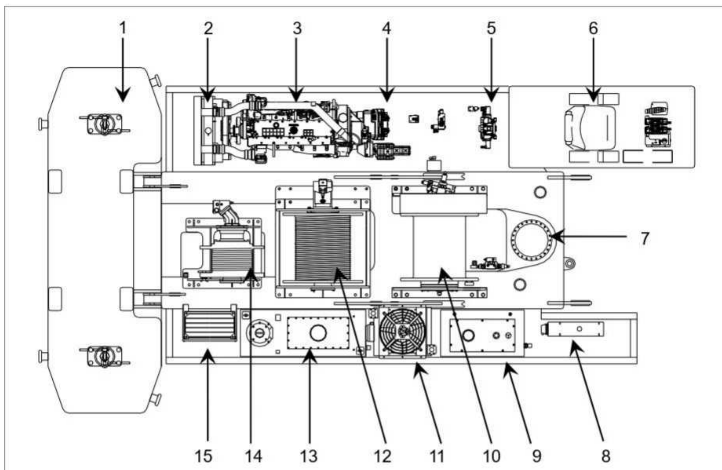
Рисунок 2-4 Размещение элементов на поворотной платформе
