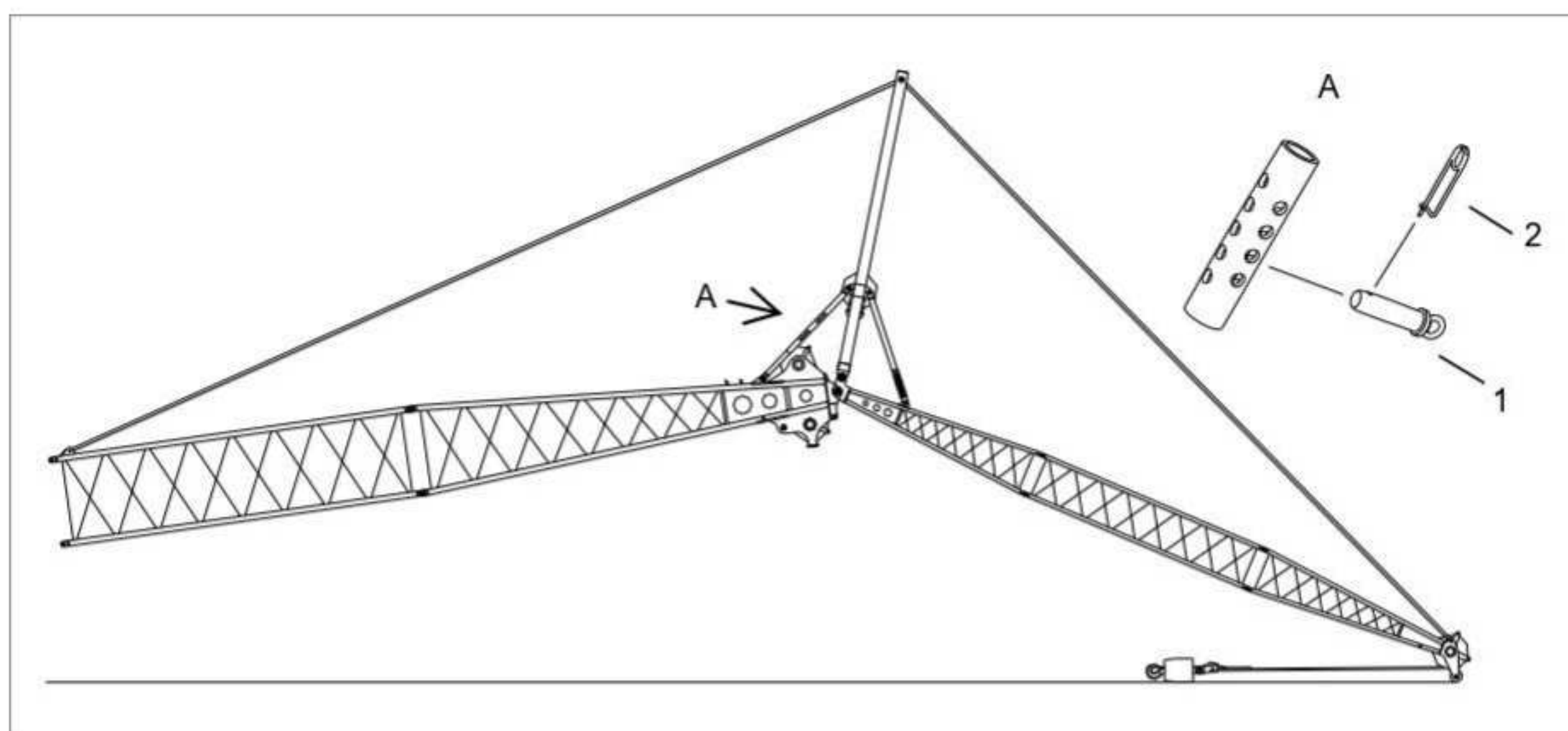
Рисунок 5-24 Монтаж каната и крюковой подвески
