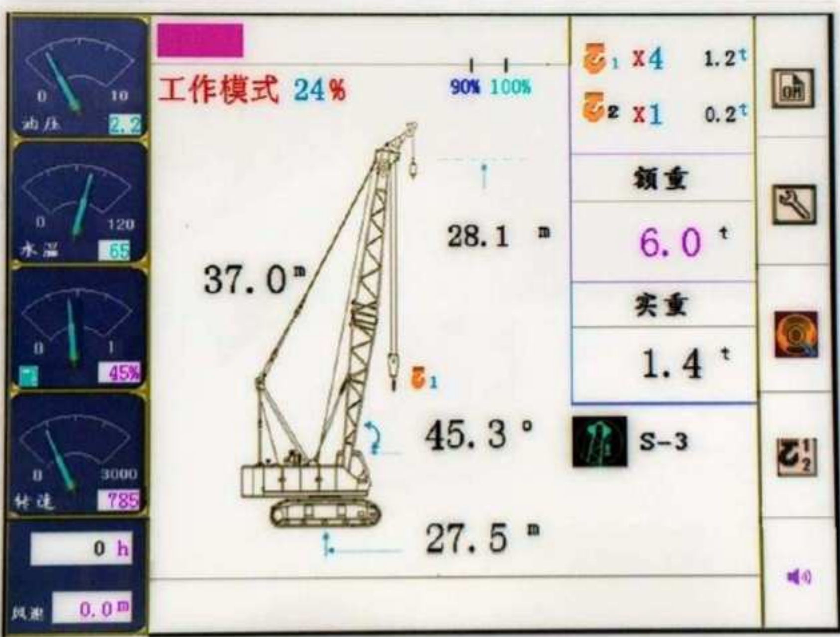
Рисунок 4-8 Главный экран дисплея ограничителя грузовой момент
