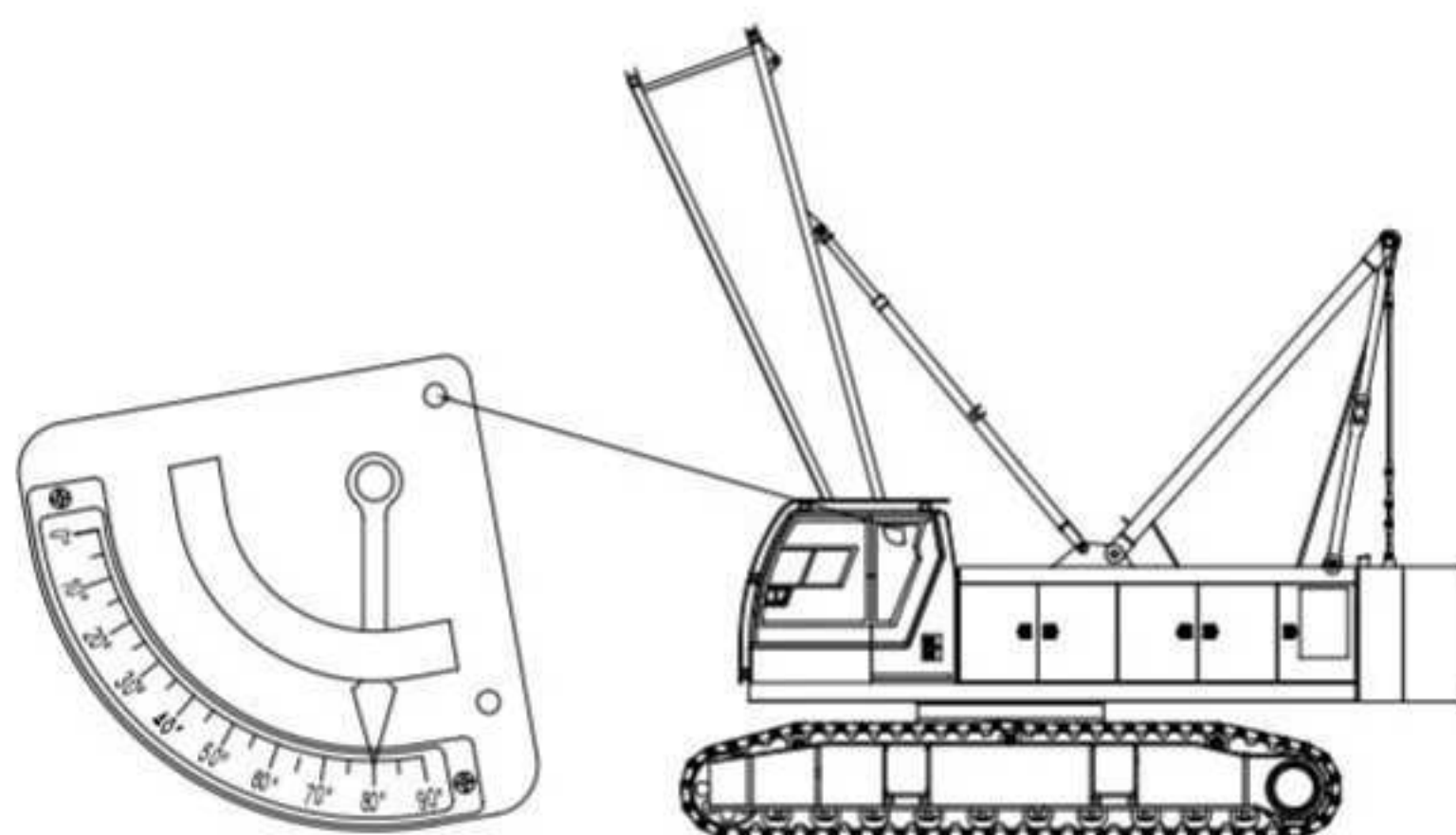
Рисунок 4-24 Место расположения указателя угла наклона стрелы
