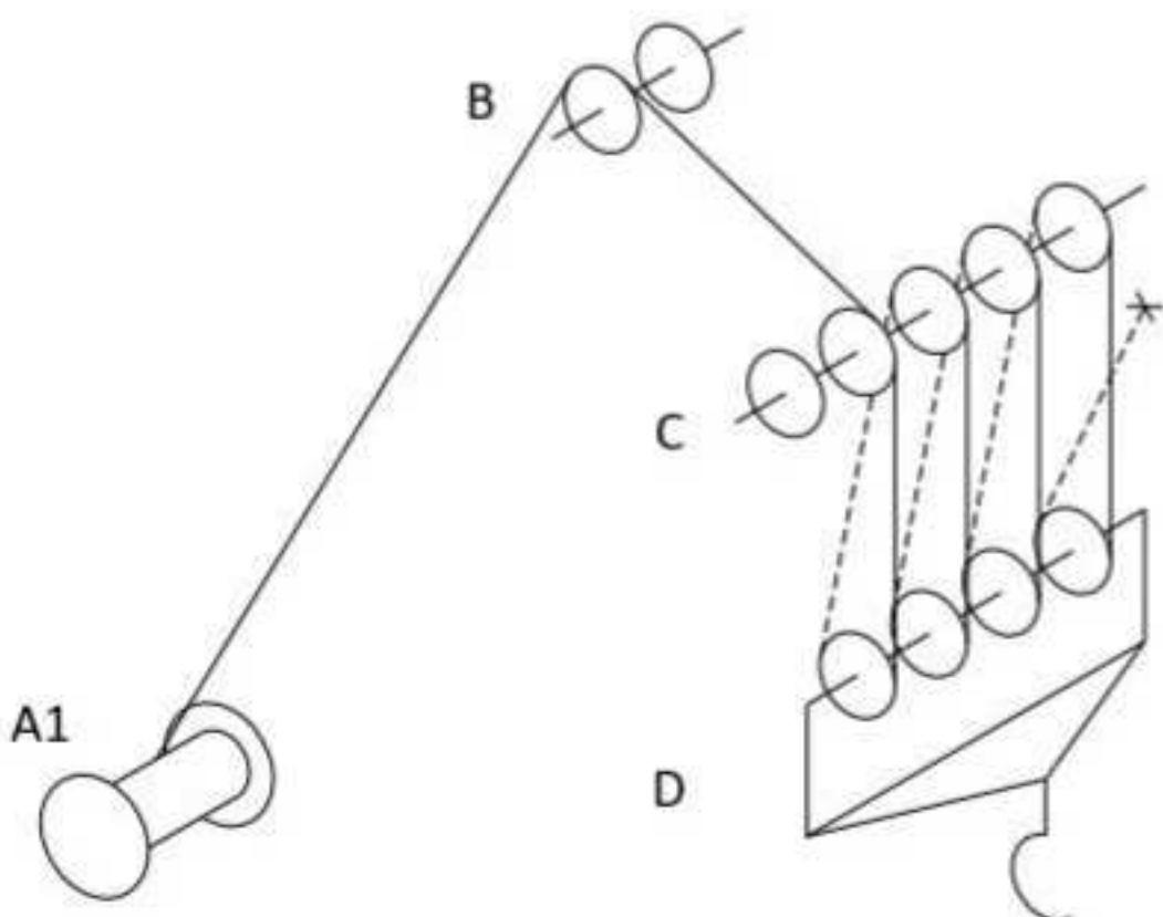
Рисунок 4-39 Схема запасовки каната (крюковая подвеска 80 т, кратность запасовки 8)
