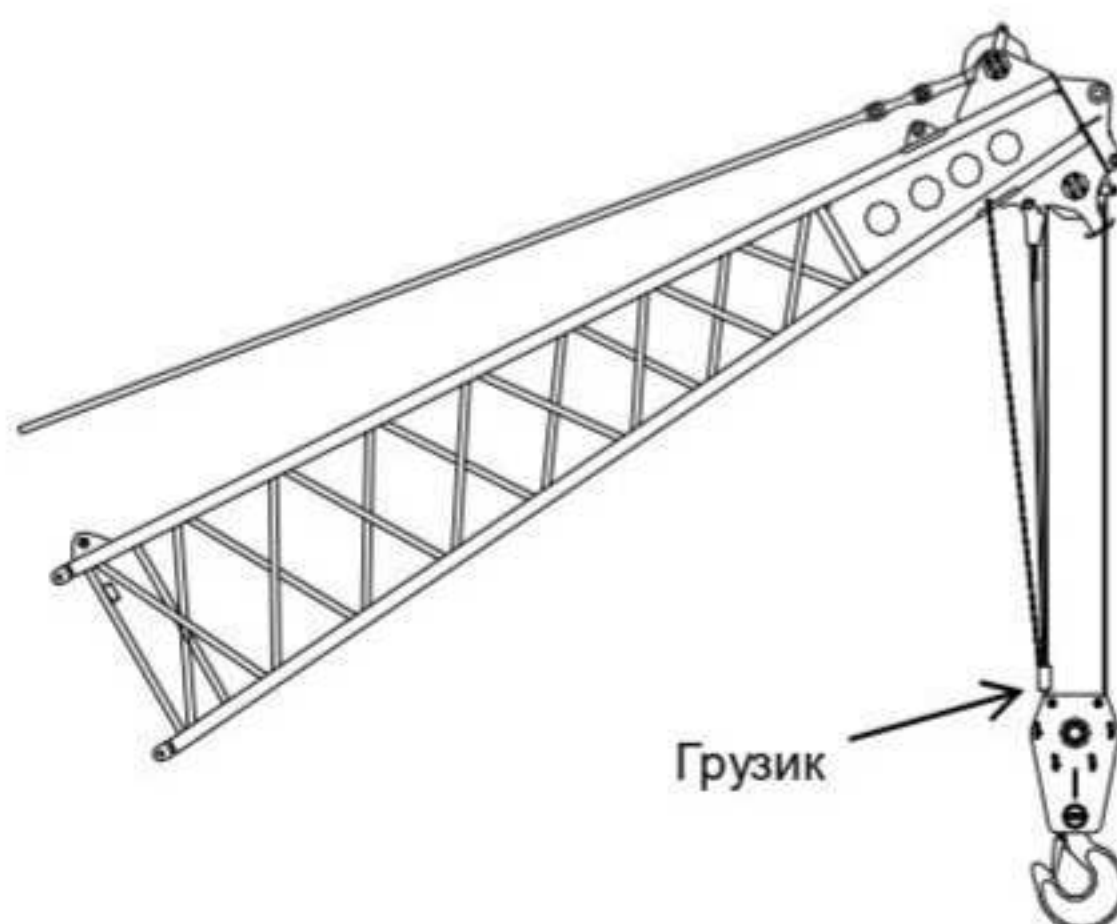
Рисунок 4-26 Ограничитель высоты подъема крюка
