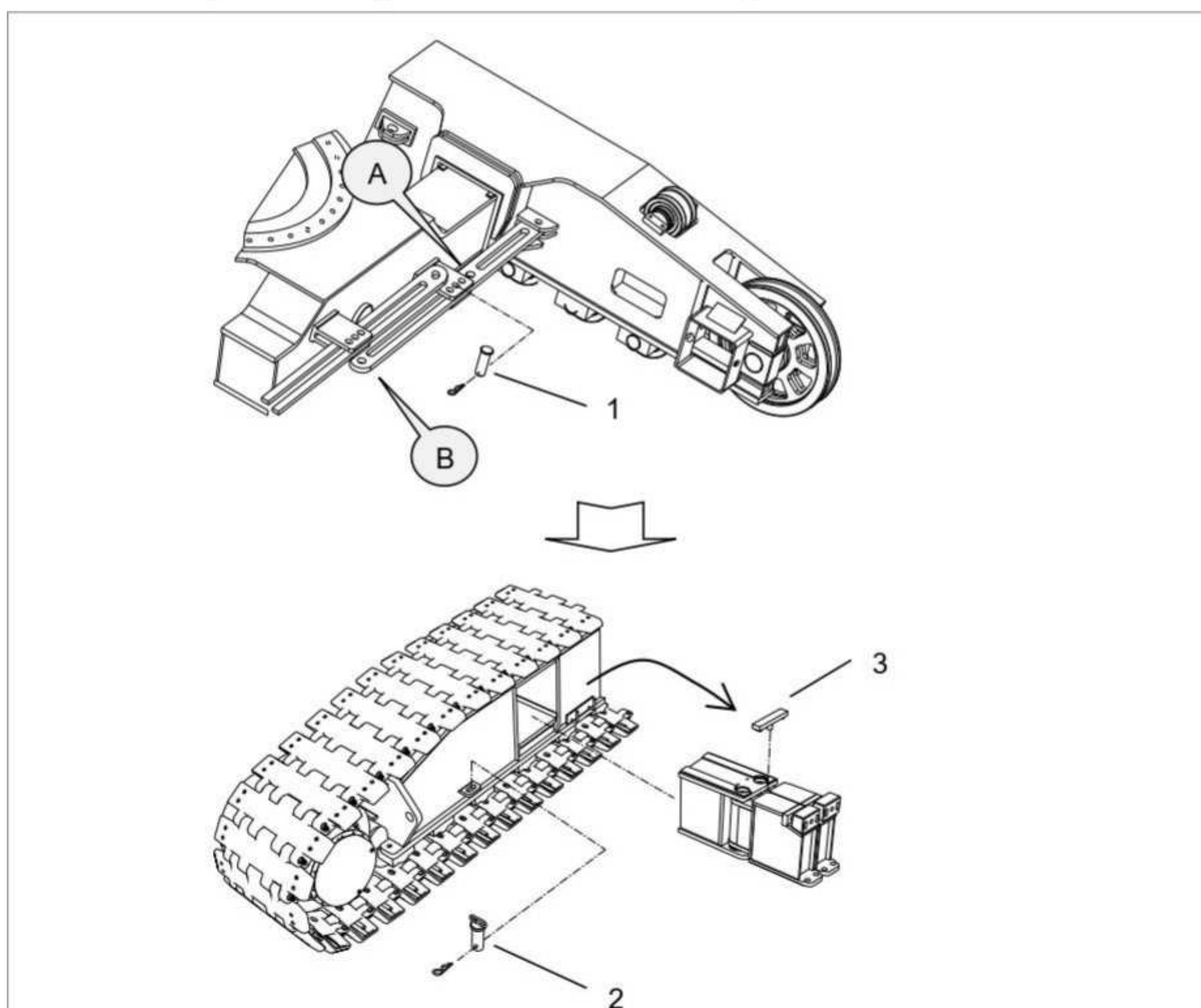
Рисунок 5-3 Подготовительные работы перед выдвижением гусеничных тележек
