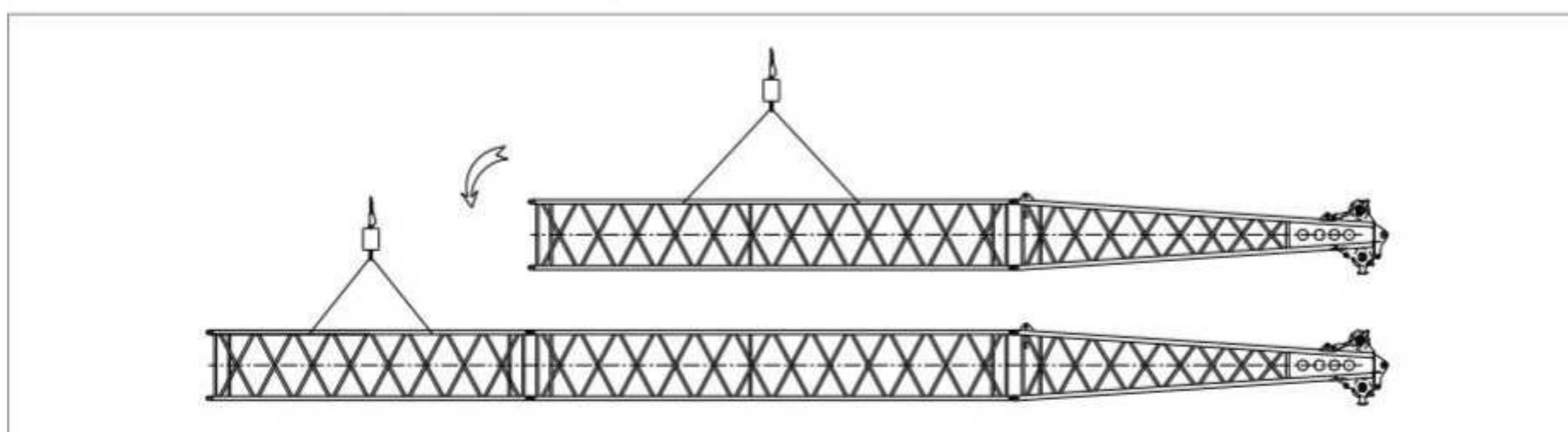
Рисунок 5-12 Предварительная сборка стрелы
