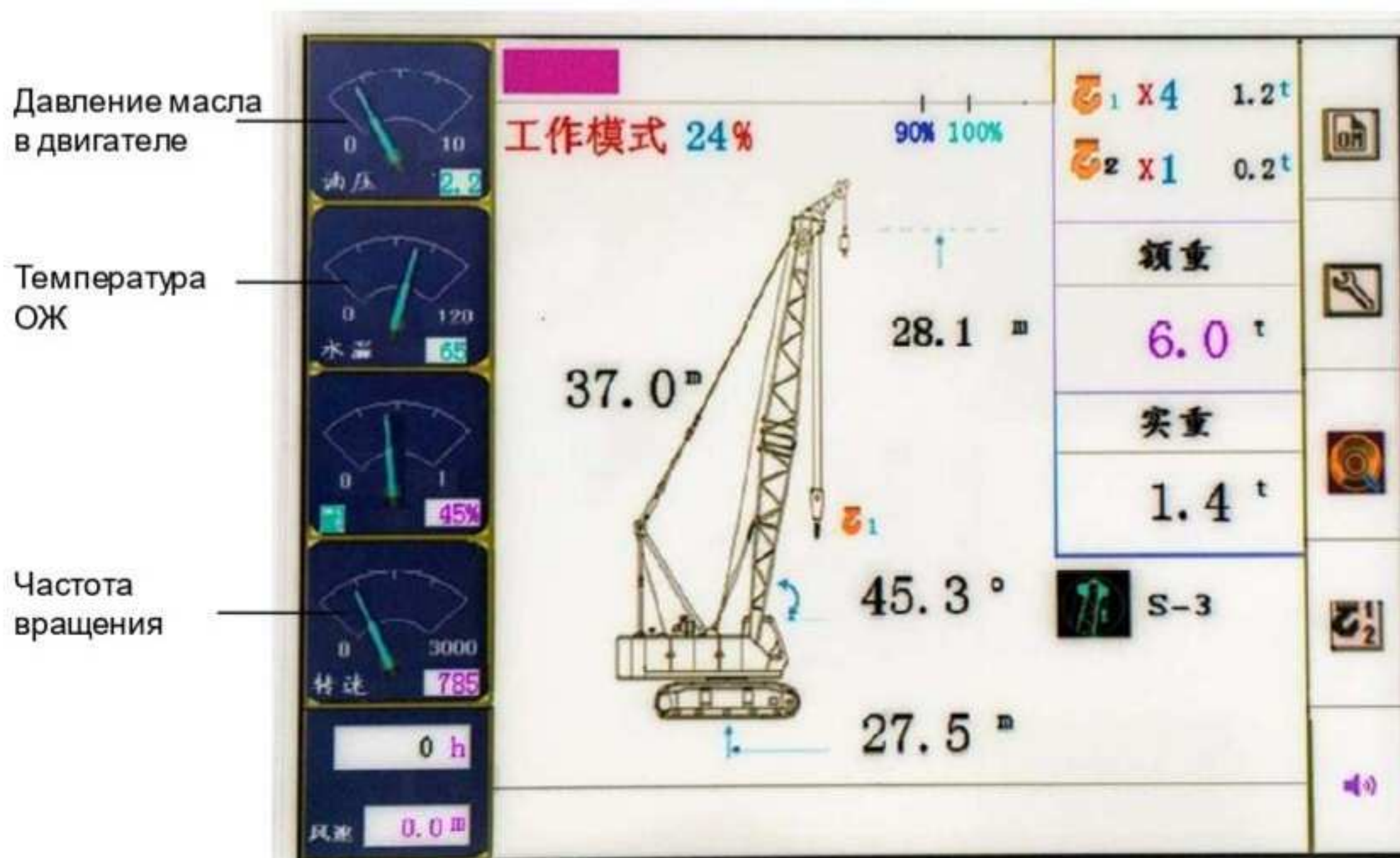
Рисунок 4-22 Проверка параметров двигателя
