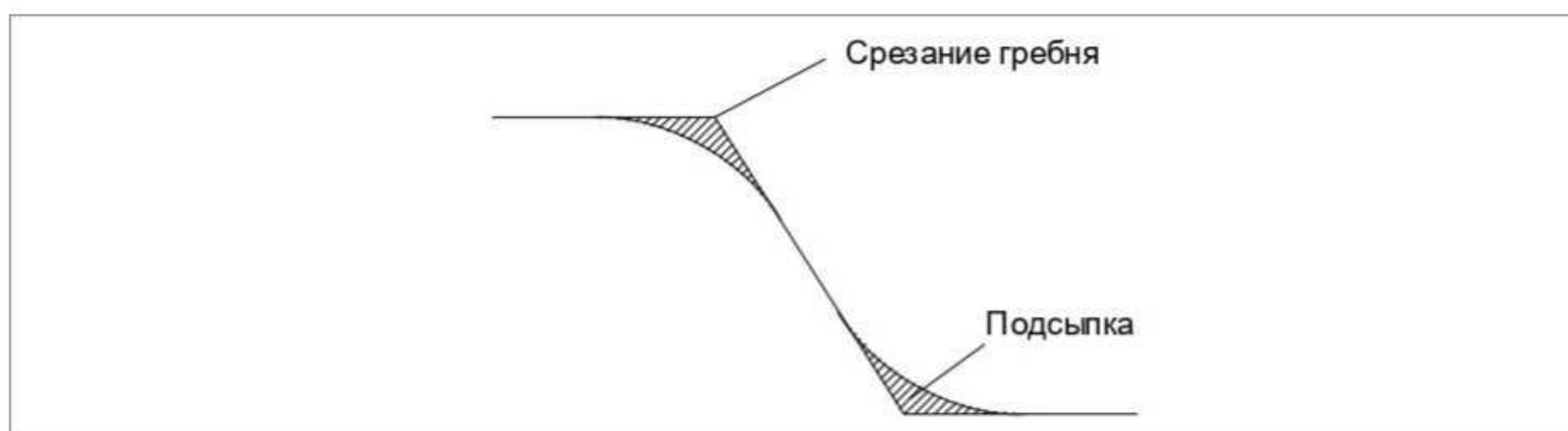
Рисунок 4-29 Схема выравнивания участка на склонах
