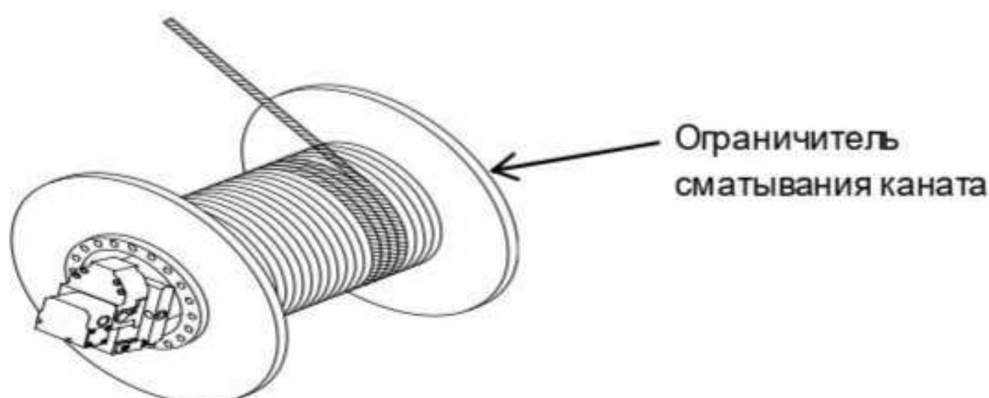
Рисунок 4-25 Ограничитель сматывания каната
