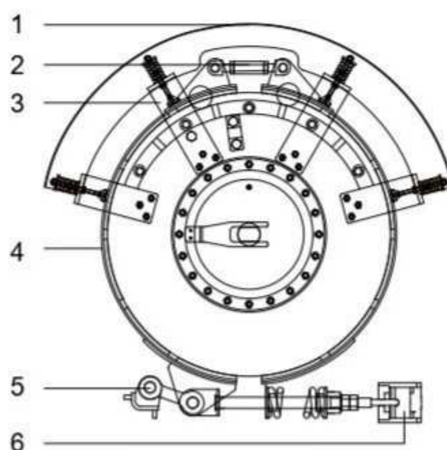
Рисунок 4-31 Ленточный тормоз лебедки со свободным спуском
